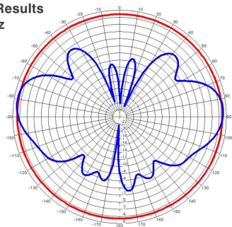
Actual Test Results 1850-1990 MHz Typical
